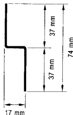
Z-Profil
